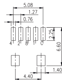
P.C.B. LAYOUT
